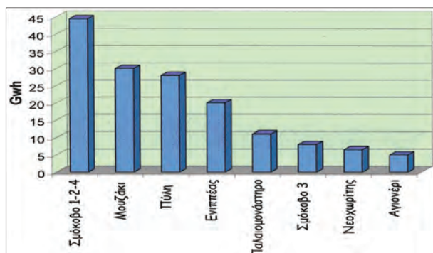
Σχήμα 4 : Μέση ετήσια παραγωγή ενέργειας νέων ταμιευτήρων Θεσσαλίας
