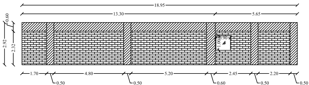
βόρεια όψη
