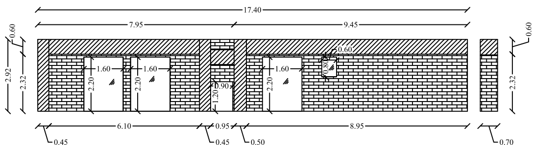
δυτική όψη
